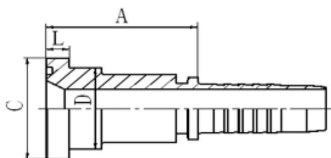
87312 SAE FLANGE 3000 PSI
