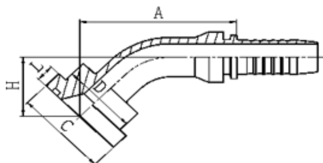
87341 45° SAE FLANGE 3000 PSI
