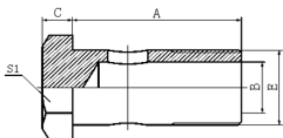
700M METRIC BOLT DIN 7643
