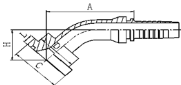
87342 45° SAE FLANGE 3000 PSI
