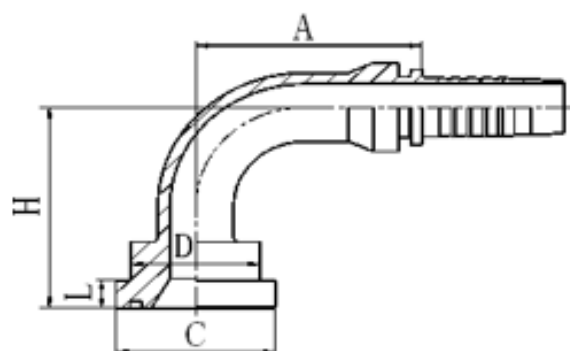
87392 90° SAE FLANGE 3000 PSI
